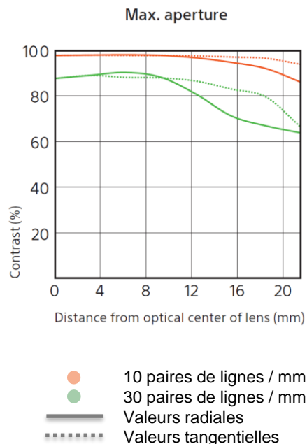
Courbes MTF : fréquence spatiale
